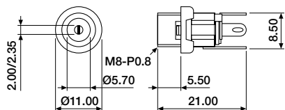
DCJ-55PM-4210/4250
