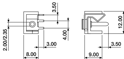
DCJ-55DS-3210/3250
