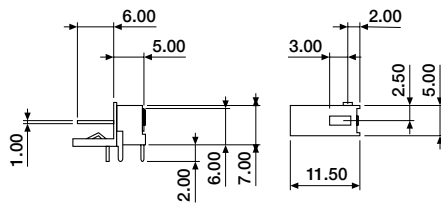
DCJ-30DS-1110
