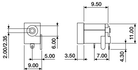
DCJ-55DS-1210/1250
